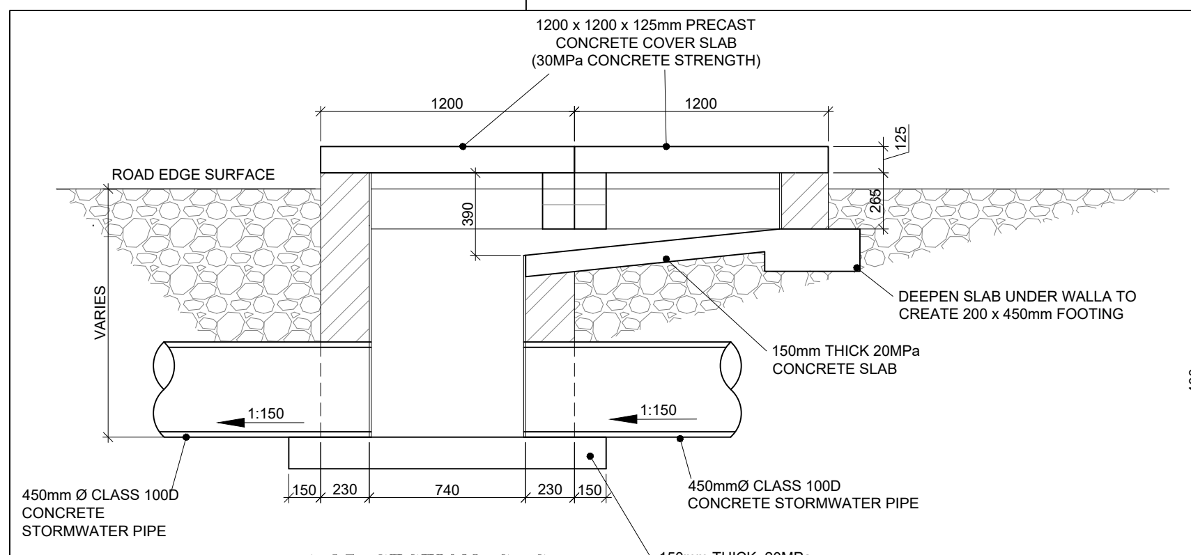
1:25 SECTION G-G
