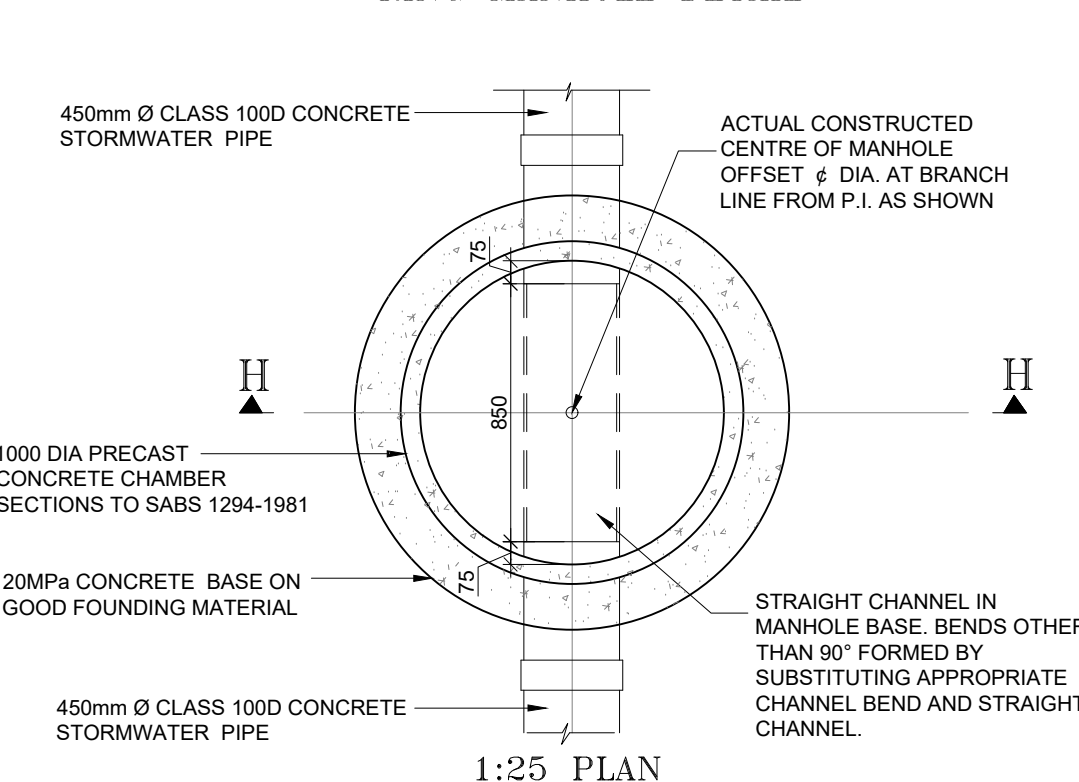
1:25 PLAN
