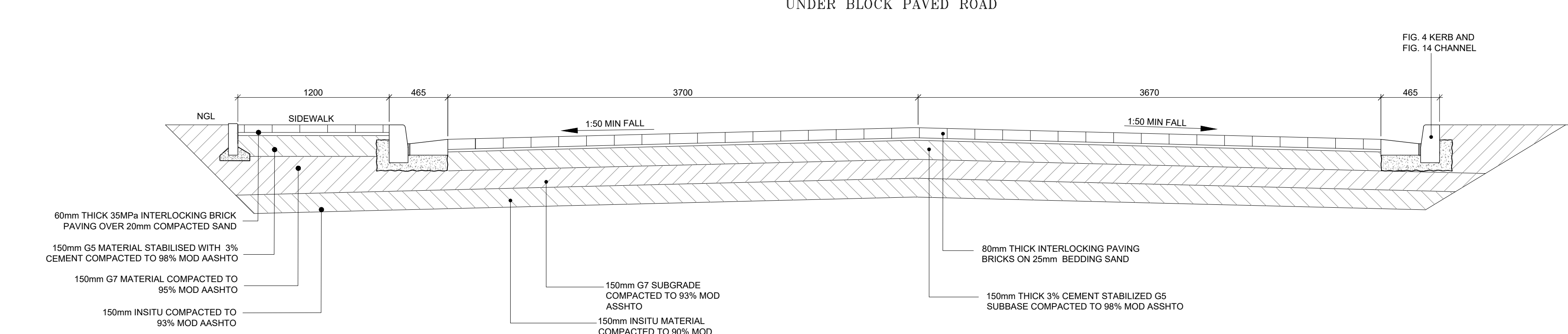
1:25 SECTION
