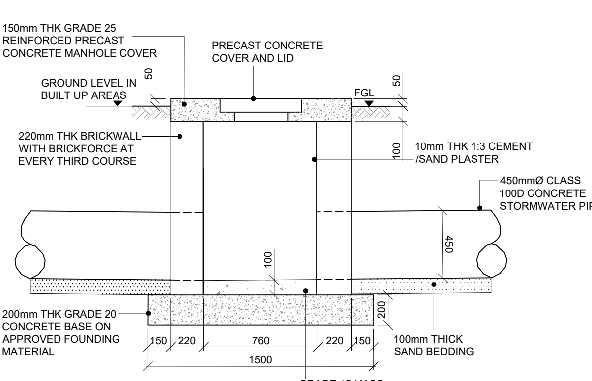
1:25 SECTION A-A
