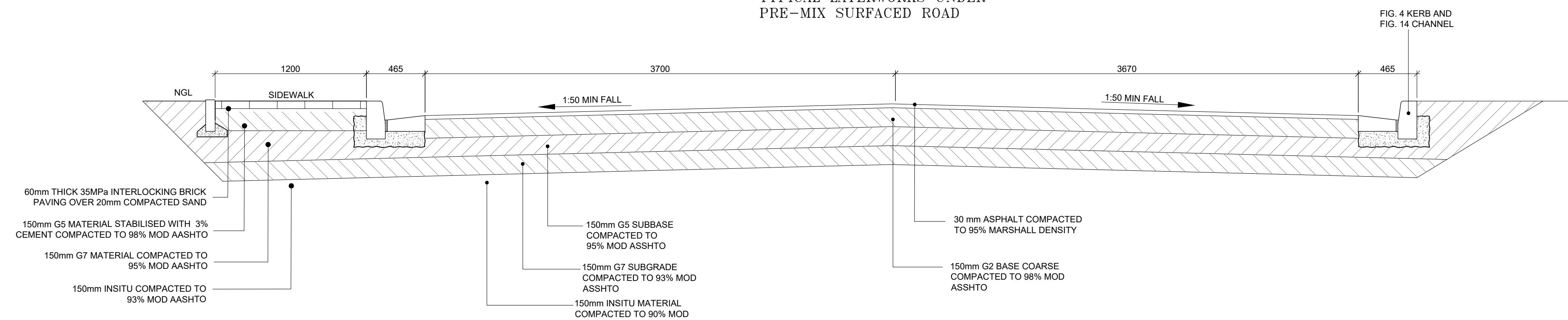
1:25 SECTION
