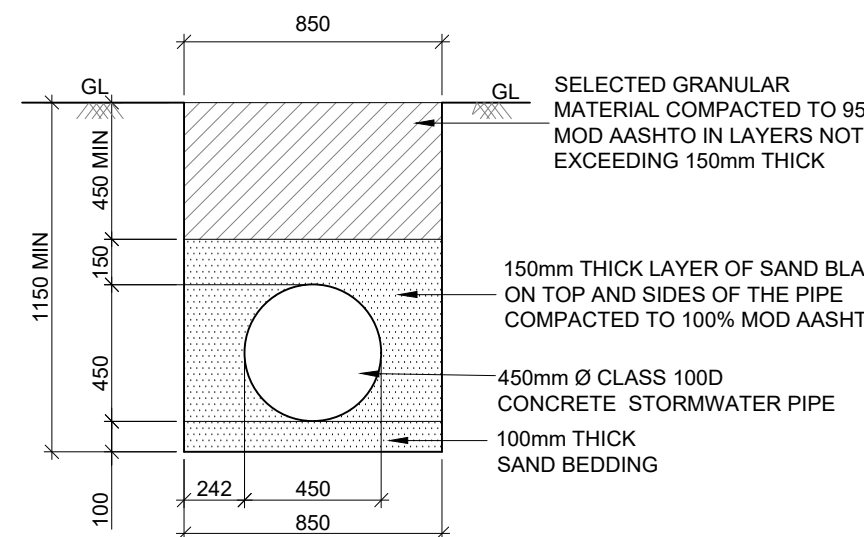
1:25 SECTION
